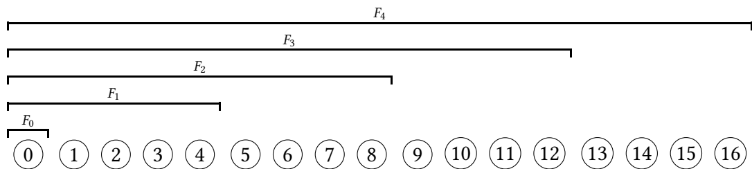
Figura 5.2: Representação da lista \text{edges\_by\_time} com m igual a 16. Neste caso, cada bloco tem tamanho 4 e os instantes 0, 4, 8, 12 e 16 são c_0, c_1, c_2, c_3 e c_4 , respectivamente. Assim, por exemplo, a estrutura F_3 contém todas as arestas adicionadas desde o instante 1 até o instante 12.
